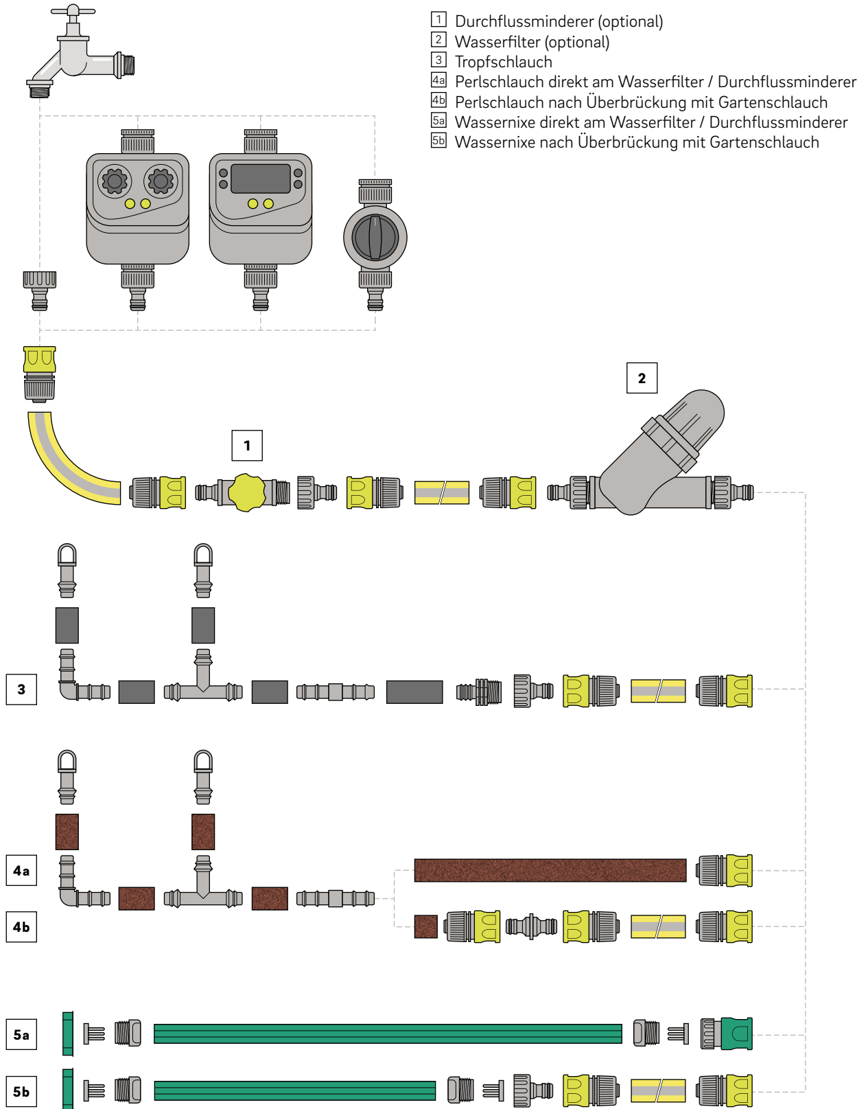
Abb. 03-1 Aufbauempfehlung Tropfschlauch, Perlschlauch und Wassernixe
