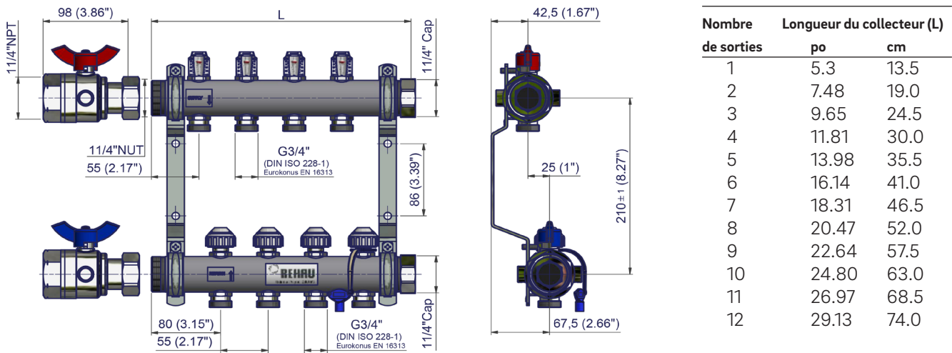
Fig. 1 : Dimensions du collecteur
