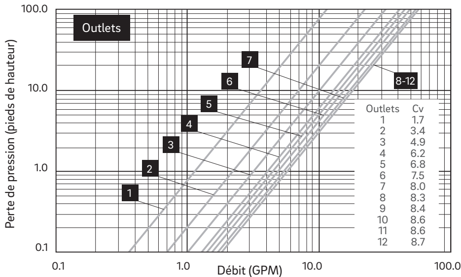
Fig. 3 : Perte de pression dans le collecteur Note : Les cases numérotées ci-dessus indiquent le nombre de sorties sur le collecteur.
