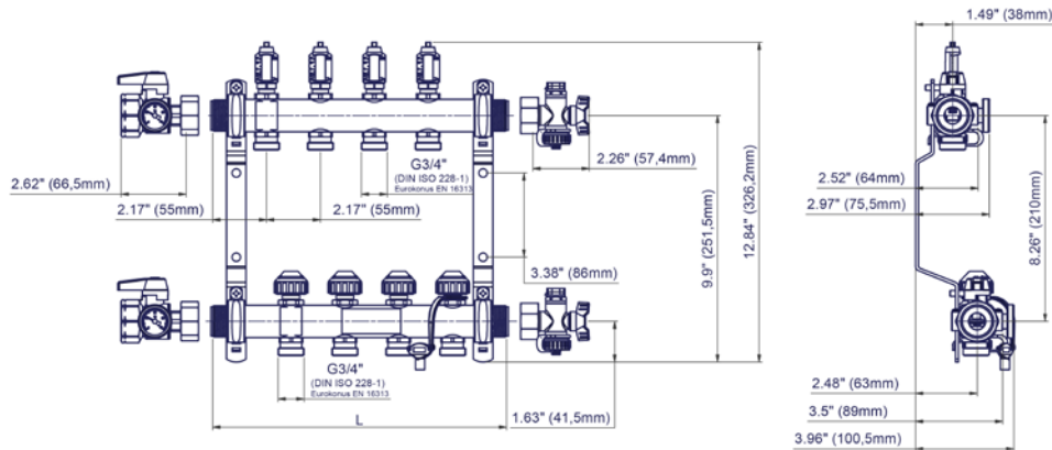
Fig. 1: Dimensiones del colector
