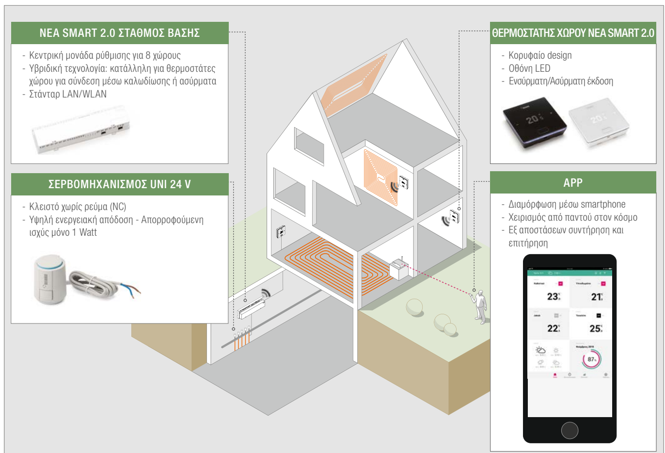
Εικ. 2-1 Σύστημα ΝΕΑ SMART 2.0
